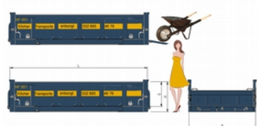
4m3 Flachmulde befahrbar (410x213x42)
