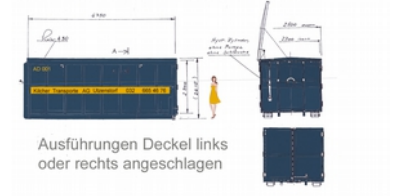
25-36m3 Abrolldeckelcont. (gegebenenfalls mit Fallsegeln ) (700x220x250)
