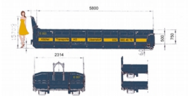
10m3 Abrollmulde
