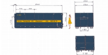
20m3 Abrollmulde
