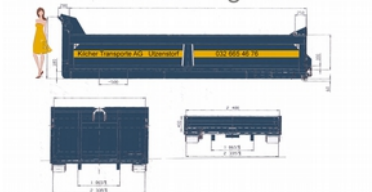
12m3 Abroll-Söringmulde
