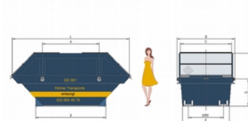
10m3 Deckelmulde beidseitig zu öffnen (430x201x170)
