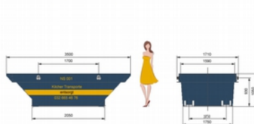
4m3 Normalmulde/ Schuttmulde (350x170x105)
