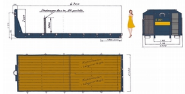
Abroll-Palette/Plattform diverse
