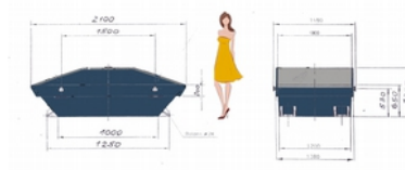
2.5m3 Mini-Deckelmulde (260x145x115)
