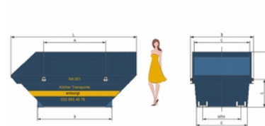
7m3 Allzweckmulde (350x170x150)
